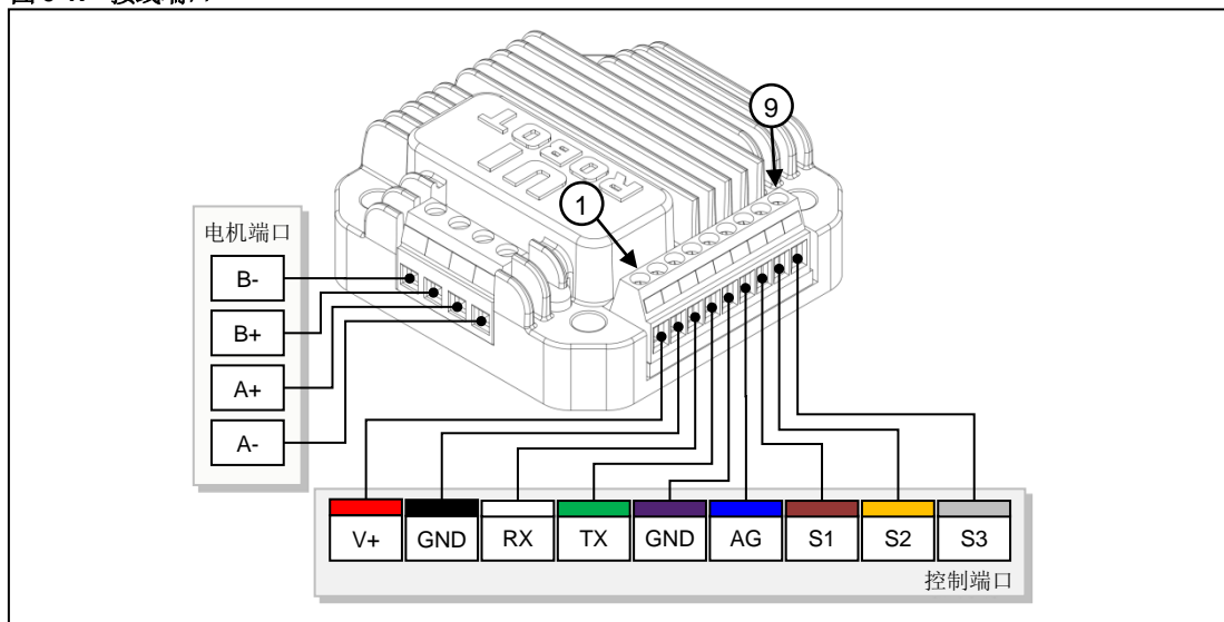
图 0-1: 接线端口
