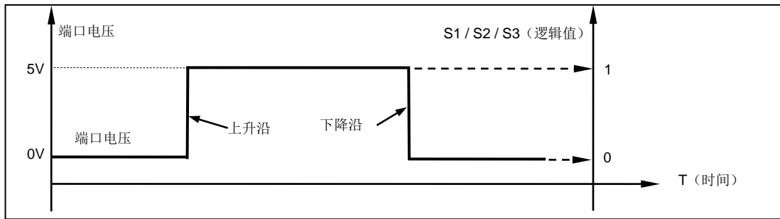
图 8-5: 传感器的上升和下降沿
