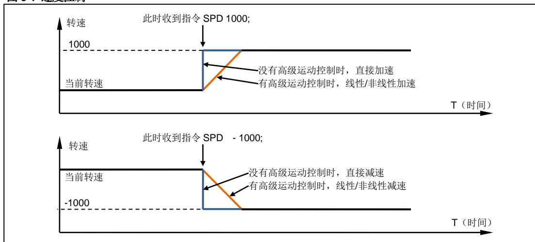
图 6-1 速度控制
