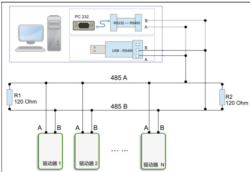
网络布局图
