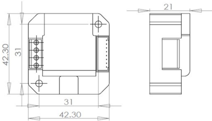
图1 UIM42RS 驱动器外形尺寸图
